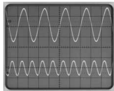
Foto: 50MHz und 100MHz Sinus-Signal mit alternierender Triggrerung
